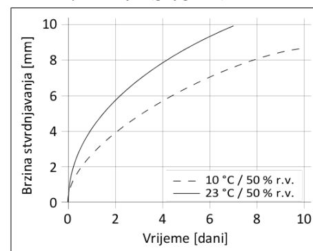
Graf 1: Prikaz utrjevanja SikaTack® DRIVE (60 min)
