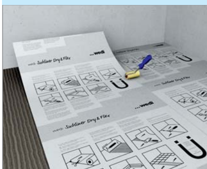
... lay membrane ...
