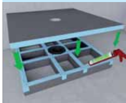
... fix Fundo Primo, done!
